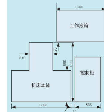
LA500 机床平面布置图:(单位:mm)
