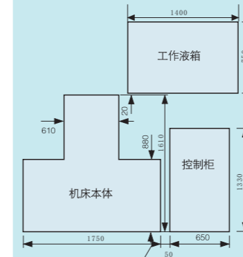
LA500 机床平面布置图:(单位:mm)
