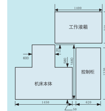
LA350 机床平面布置图:(单位:mm)
